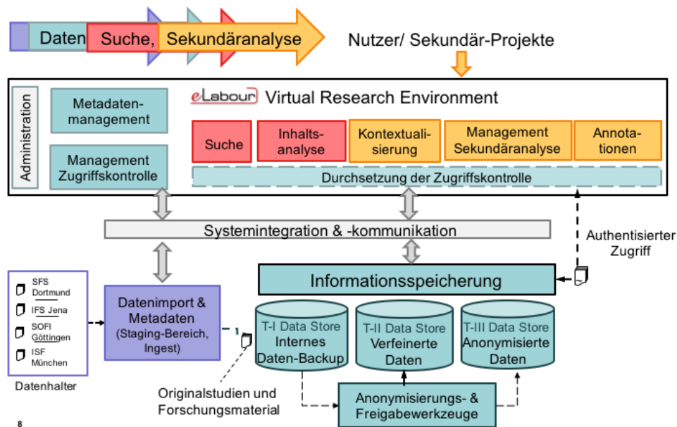
Abbildung 3: Aufbau der Forschungsinfrastruktur
